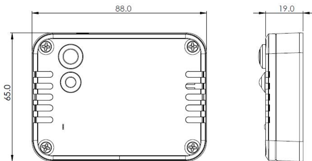
图一 主机外壳尺寸图
